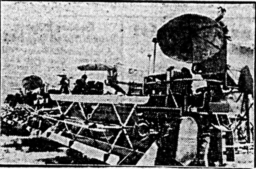
A novo-jegorevcskaja gép- és traktorállomáson vizsgálják, javítják a kolhozparaszt nagy segítőit, a gépeket.
